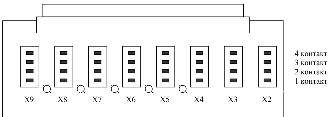
Рисунок 2. Внешний вид платы KP52.
