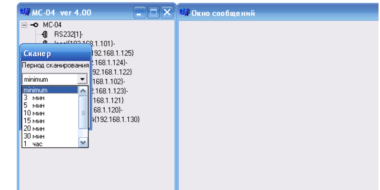
Рис.3.3. Панель управления сканером и окно сообщений
