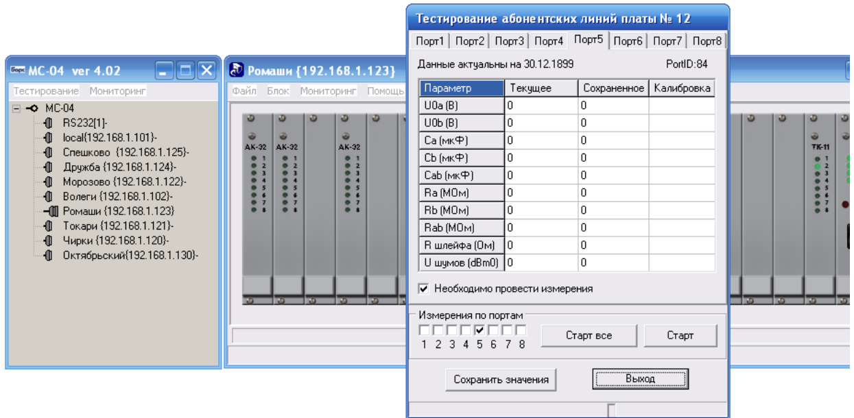
Рис 5.3 Тестирование абонентской линии.
